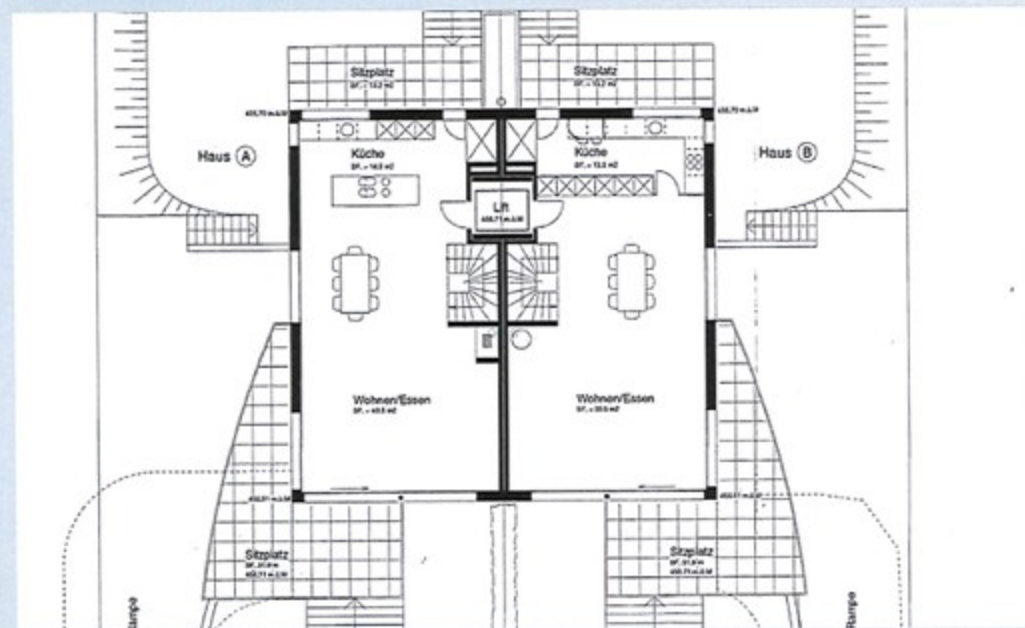
Wohngeschoss
