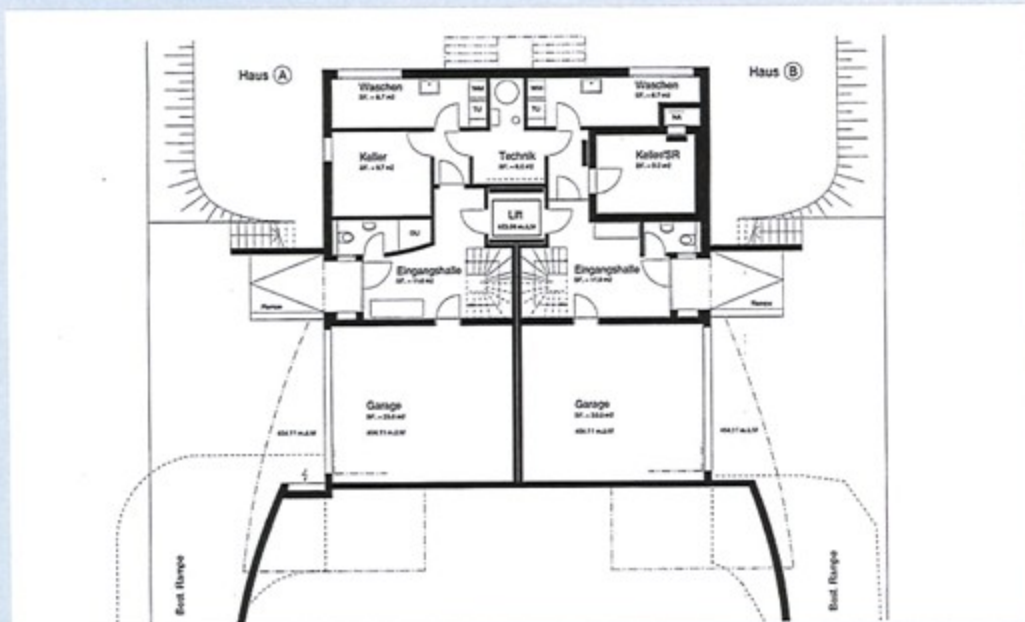
Einbaugeschoss
