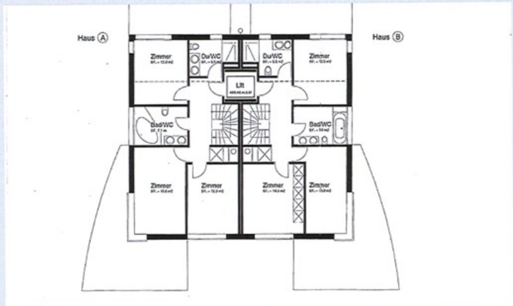
Obergeschoss
